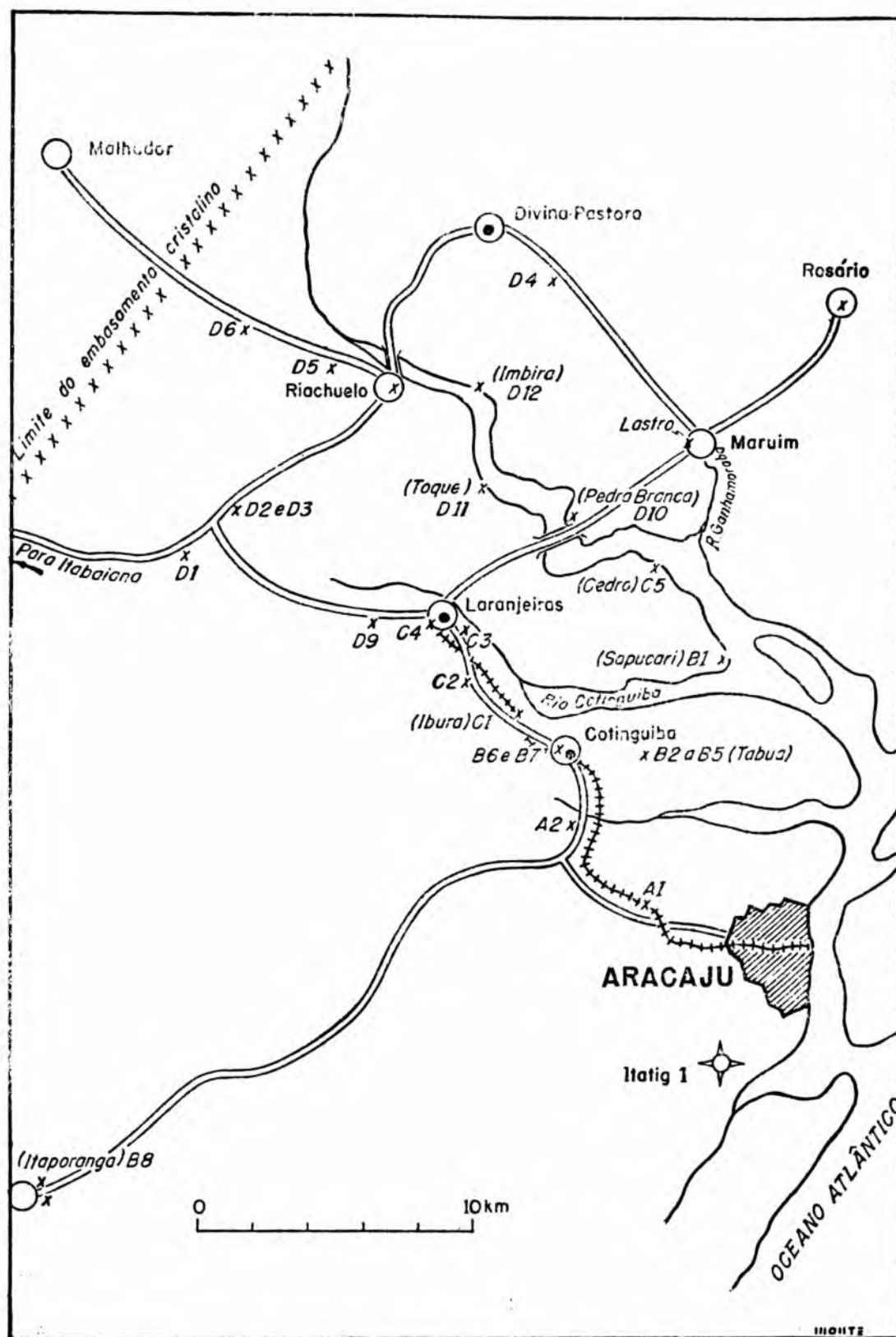
Fig. 2 — Localização das amostras coletadas. Região SW da faixa cretácea de Sergipe.
