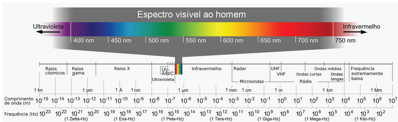
Figura 50. Espectro eletromagnético.
