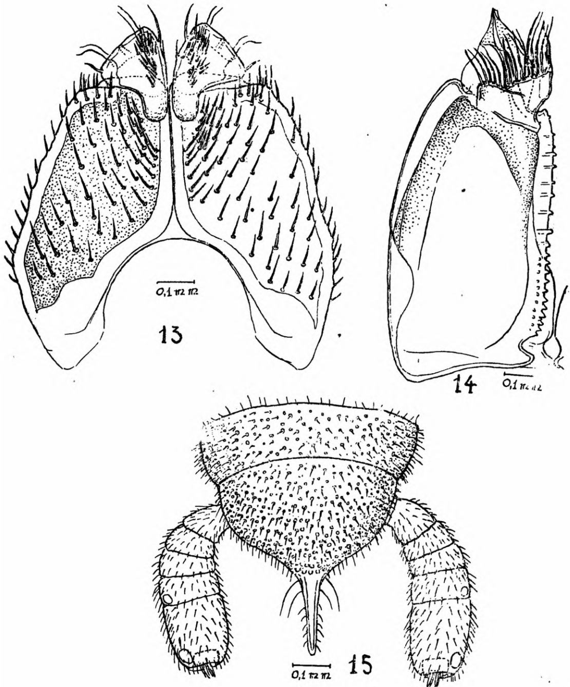
Fig. 13 Pseudonannolene urbica ; coxas e pré-fêmur do 2º par de pernas; ♂, São Paulo.
